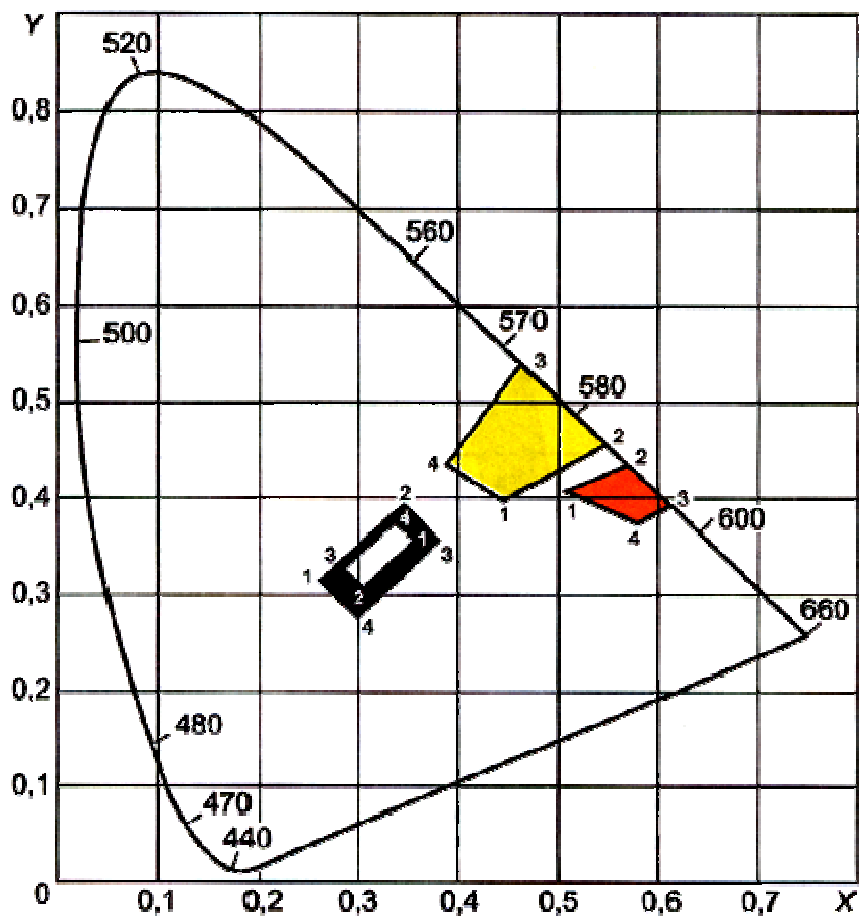
Рисунок В.1 - График цветовой области для дорожной разметки (МКО, 1931)
