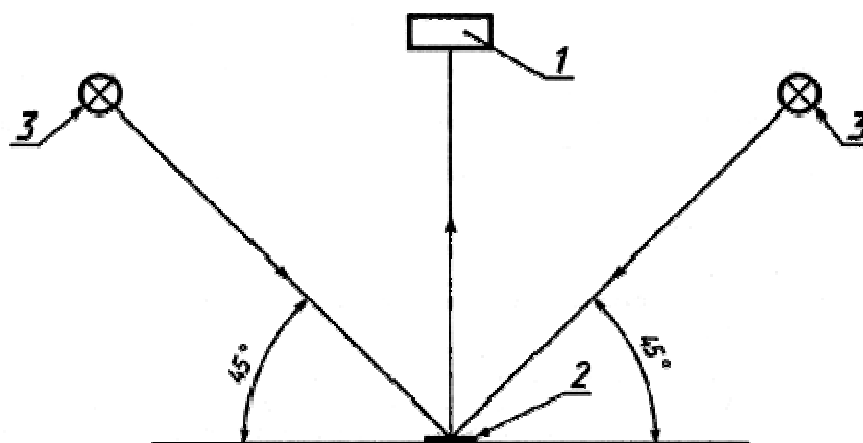
1 - спектрофотометр или колориметр; 2 - дорожная разметка; 3 - источник света
