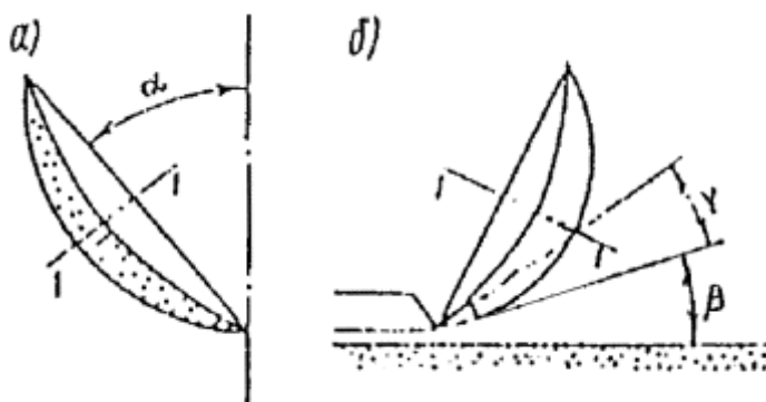
Рис. 3.6. Углы установки дискового плуга грейдера-элеватора:
