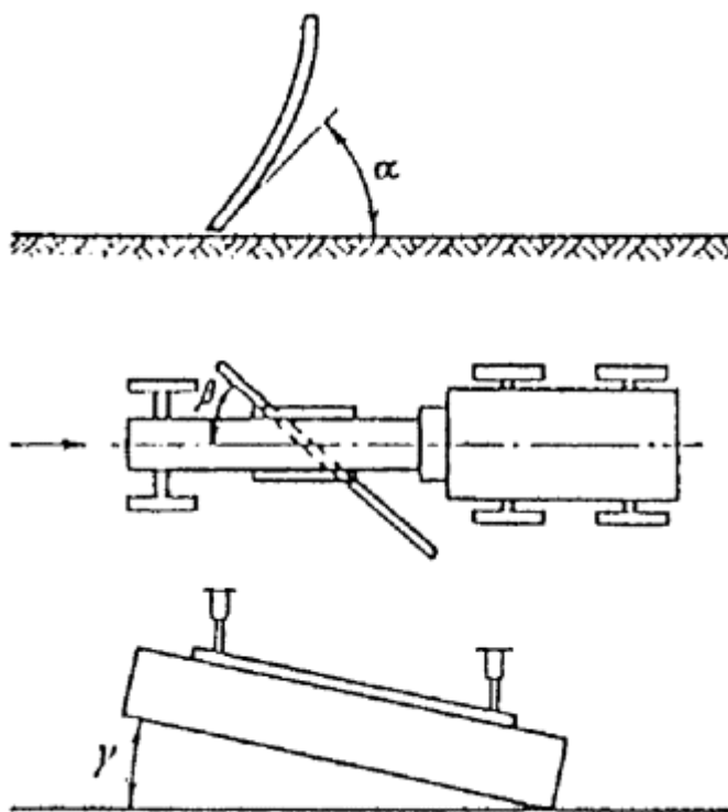
Рис. 3.5. Угли установки ножа грейдера (автогрейдера):
