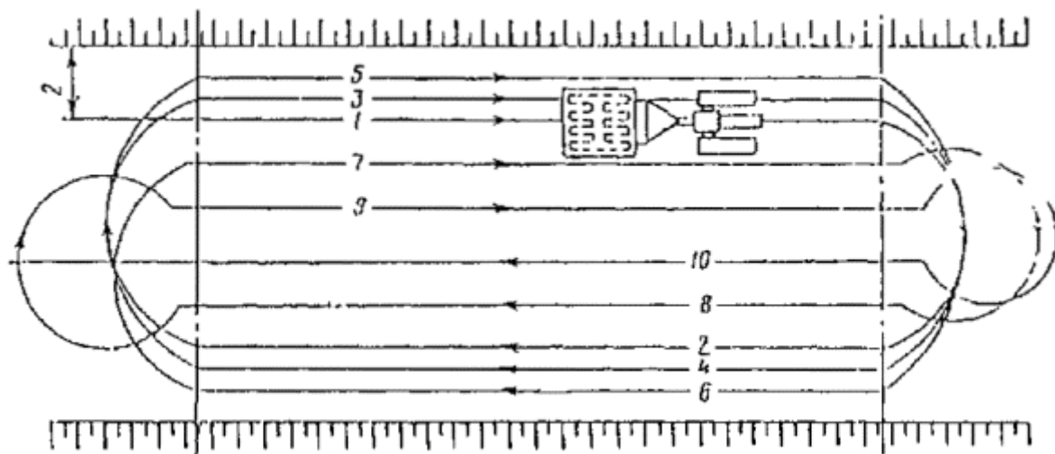
Рис. 4.2. Схема работы прицепного катка на пневматических шинах:
