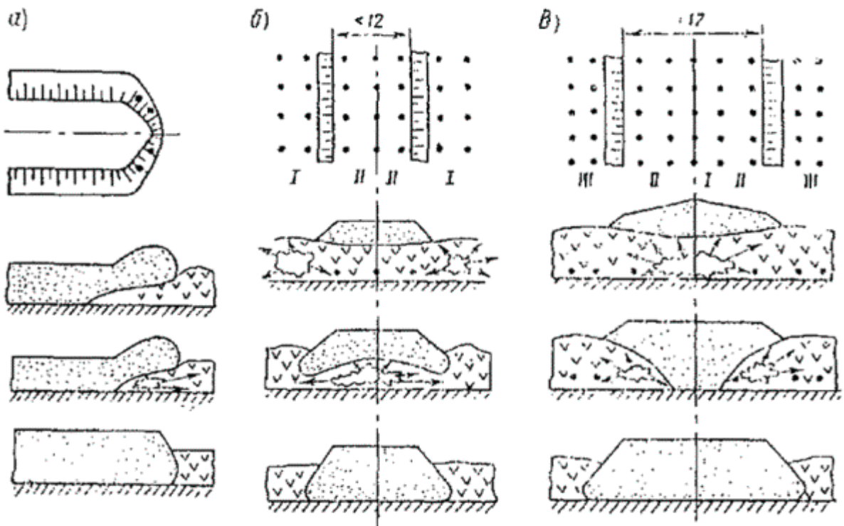
Рис. 12.5. Технологические схемы взрывного выторфовывания:
