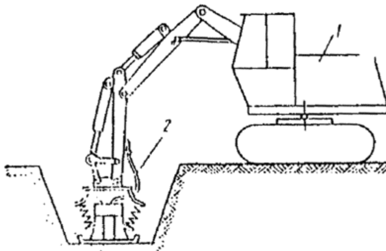
Рис. 4.7. Уплотнение грунта обратной засыпки траншеи:
