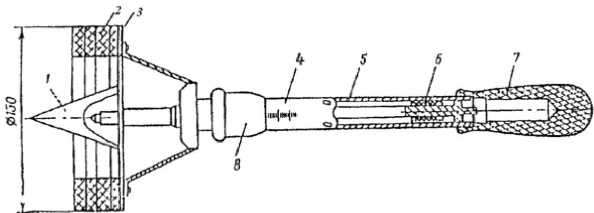
Рис. 4. Пенетромтр:
