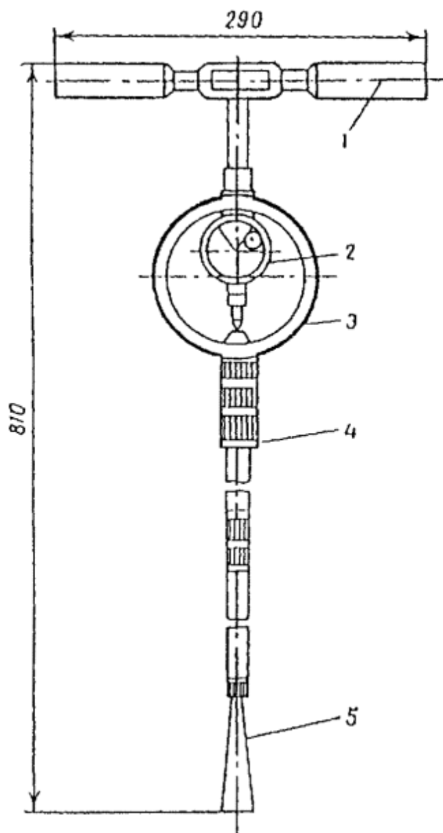
Рис. 1. Плотномер пенетрационный статического действия СП
