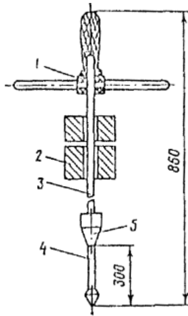
Рис. 8. Динамический плотномер:
