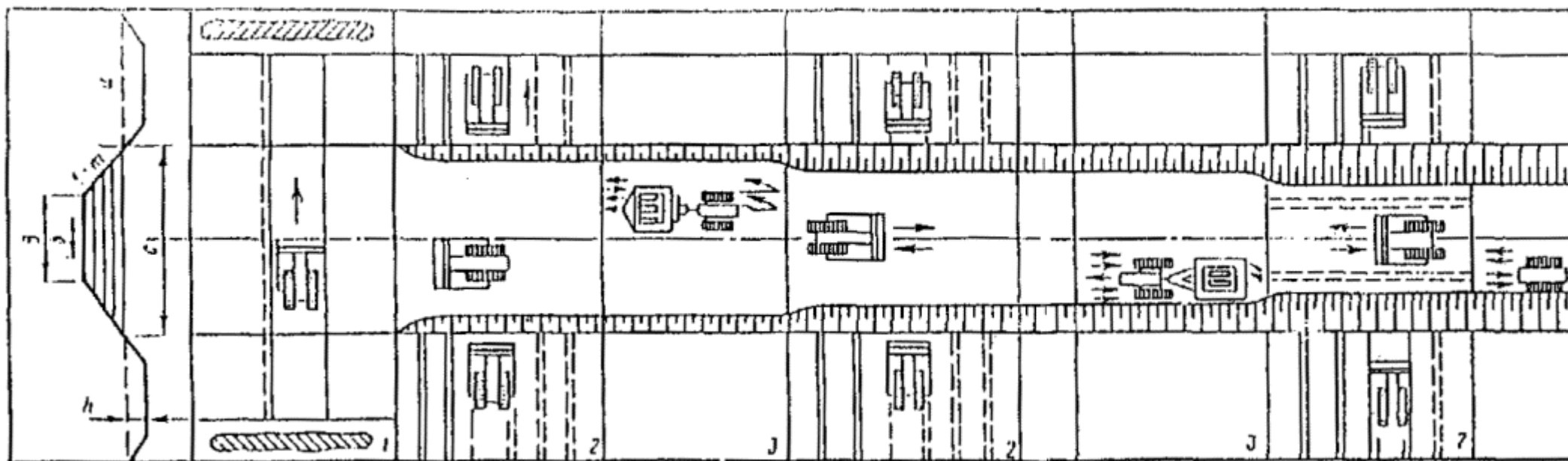
Рис. 3.7. Технологическая схема возведения насыпи из боковых резервов бульдозерами:
