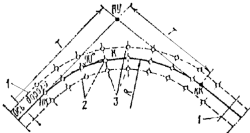
Рис. 2.3. Схема закрепления оси дороги на криволинейном участке трассы:
