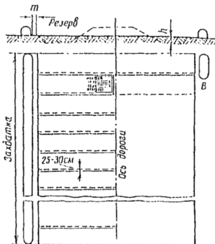
Рис. 3.2. Схема снятия плодородного слоя почвы поперечным способом на полосе шириной 30-10 м и более:
