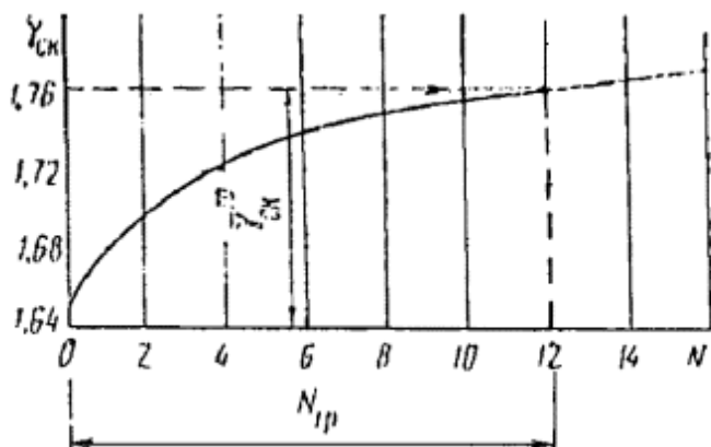
Рис. 2. График зависимости плотности сухого грунта от количества проходов катка по одному следу \bar{\gamma}_{сж} = f(N)
