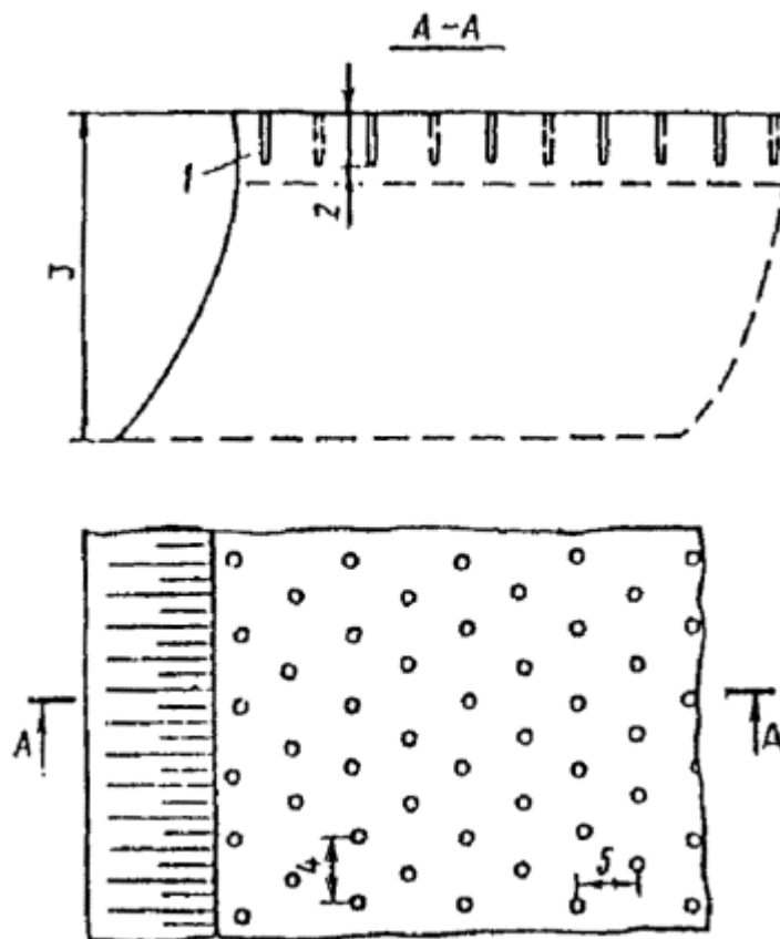
Рис. 9.5. Схема расположения шпуров (скважин при рыхлении мерзлых грунтов):
