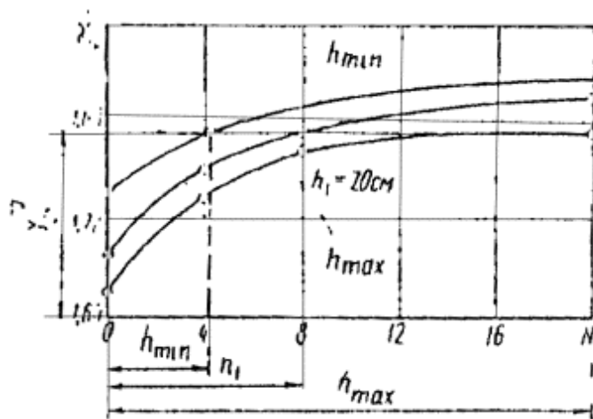
Рис. 4. Зависимость плотности сухого грунта от количества проходов катка по одному следу \bar{\gamma}_{\text{сух}} = f(N)_{\text{ж}} ; для различных значений толщины слоя грунта в интервале ( h_{\text{min}} - h_{\text{max}} )
