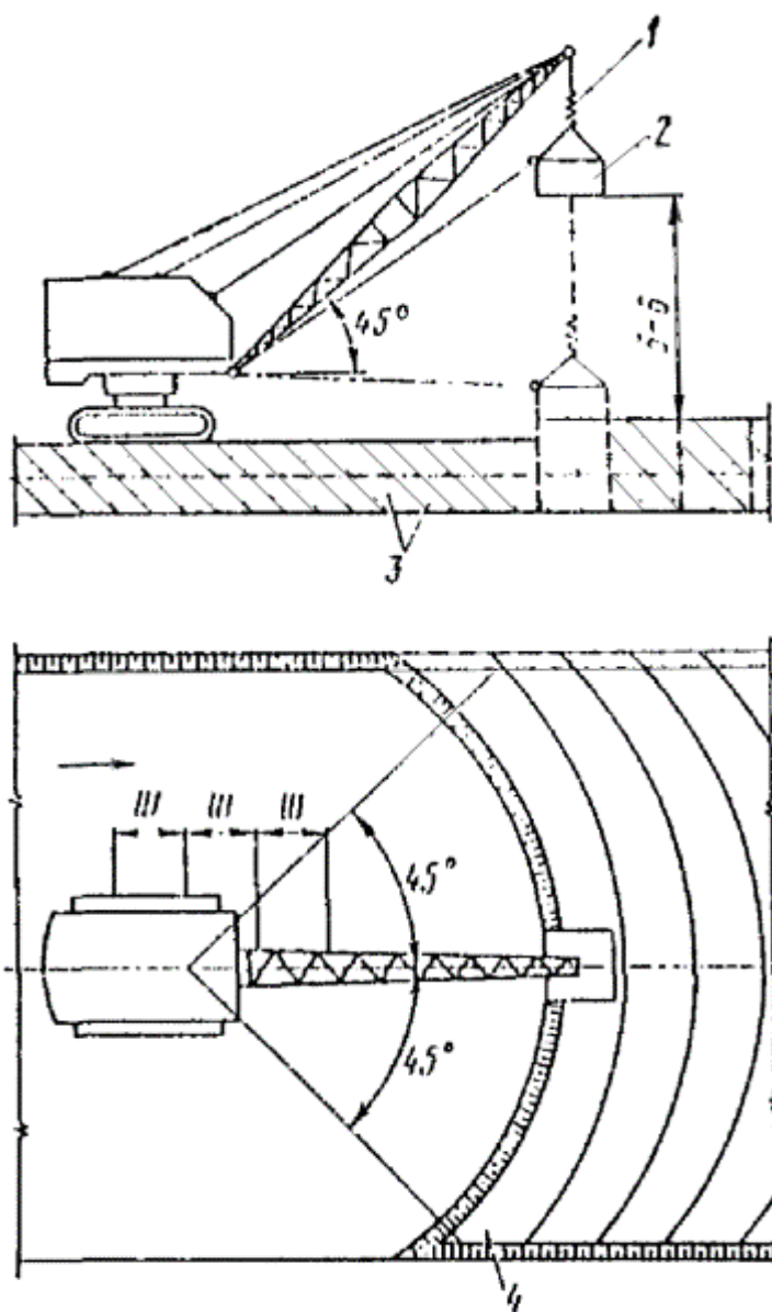
Рис. 4.4. Схема работы тяжелой (масса 12-15 т) трамбующей плиты, подвешенной к стреле экскаватора:
