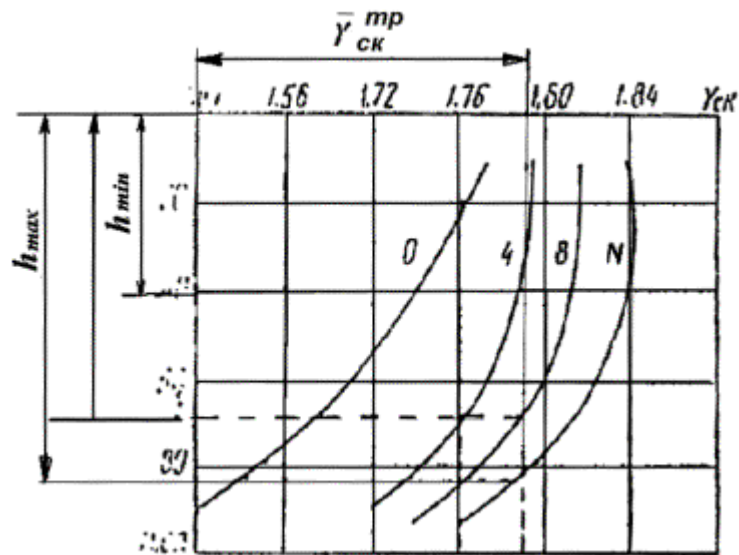
Рис. 3. Зависимость плотности сухого грунта по толщине пробного слоя от количества проходов катка по одному следу \bar{\gamma}_{ск} = f(h_{сп}, N) .
