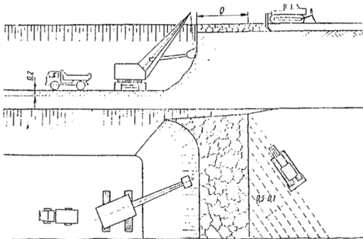
Рис. 9.3. Схема разработки грунта в зимних условиях экскаватором, оборудованным прямой лопатой, с применением рыхлителя для разрушения мерзлого слоя:
