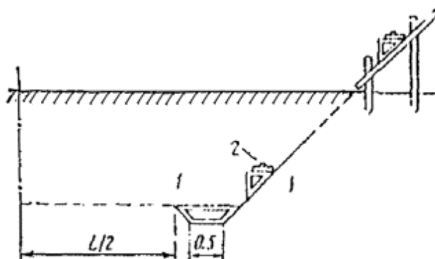
Рис. 3.10. Разбивка выемки:
